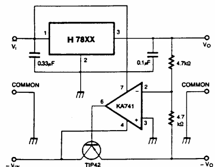
图 10、跟踪稳压器
