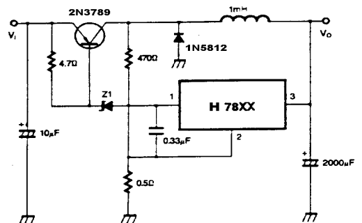
图 13、开关稳压器
